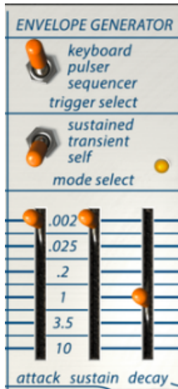
Réglages pour l'Envelope Generator
