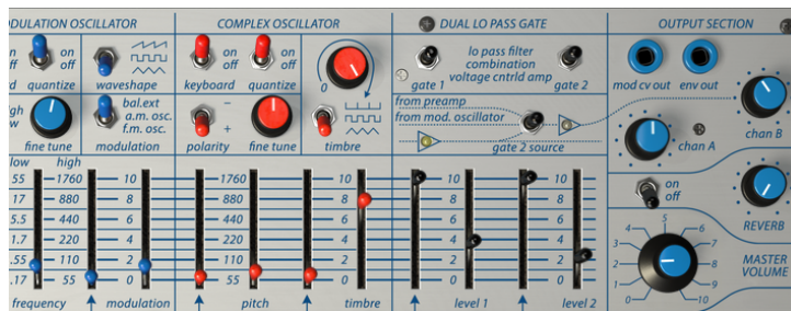
Les deux oscillateurs routés sur le Lo Pass Gate
