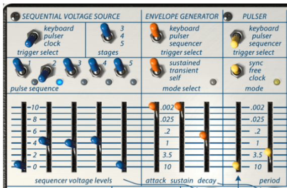
La Sequential Voltage Source déclenchée par le Pulser
