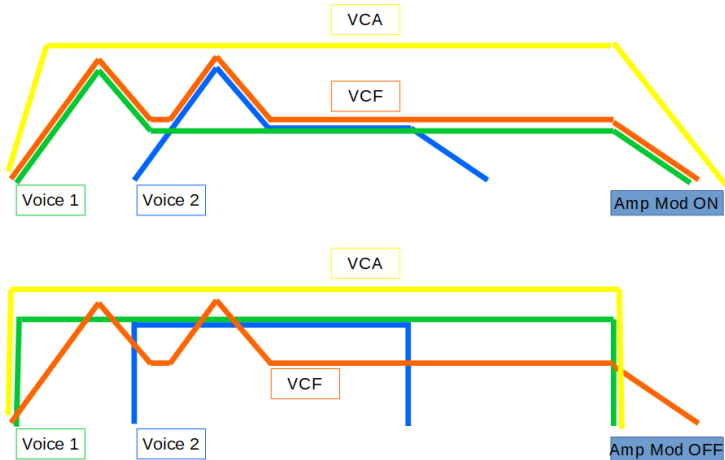
El flujo de señal de MicroFreak.
