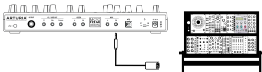
MIDIでモジュラーと接続
